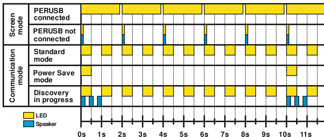
Obr. 3 Signalizace režimů a stavů brány pomocí LED a Speakeru
