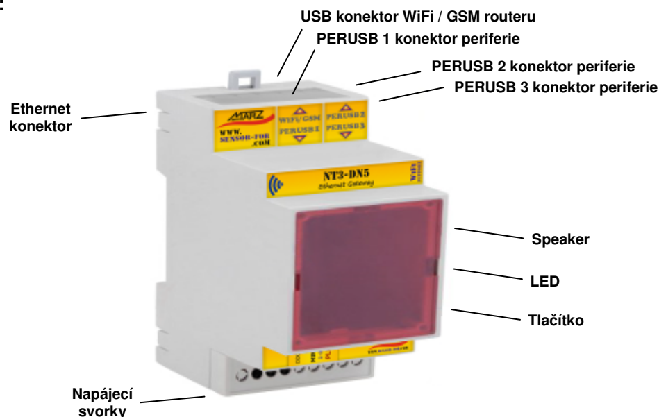
Obr. 2 NT3-DN5, popis zadní a přední strany
