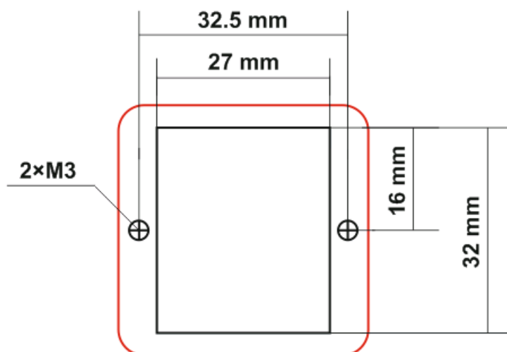
Obr. 1.1 Montážní výkres
