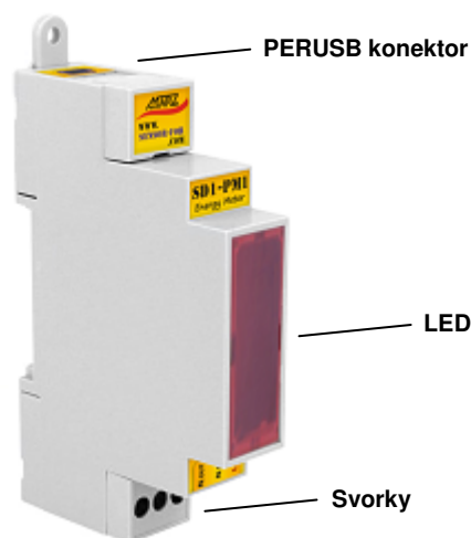
Obr. 3 Popis modulu SD1-PM1
