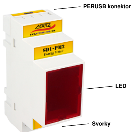
Obr. 3 Popis modulu SD1-PM2
