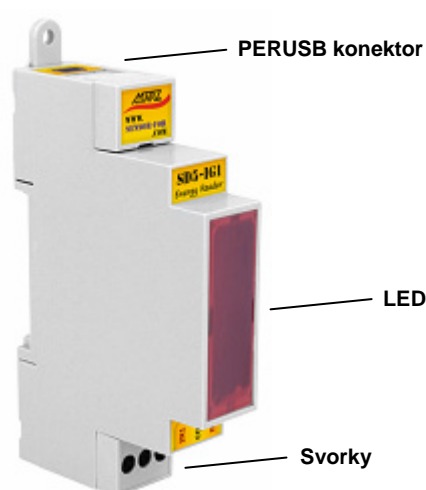
Obr. 3 Popis modulu SD5-IG1
