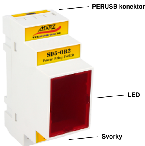
Obr. 3 Popis modulu SD5-OR2
