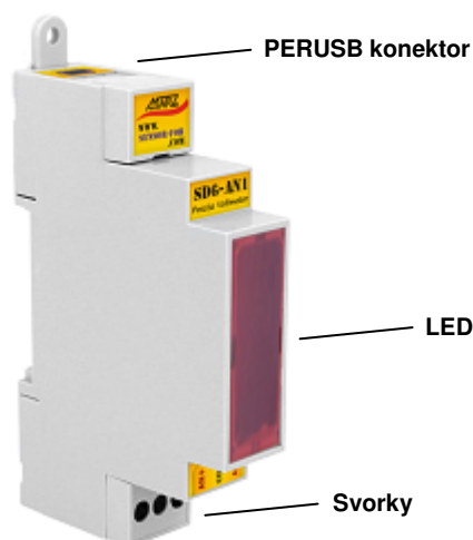
Obr. 3 Popis modulu SD6-AN1
