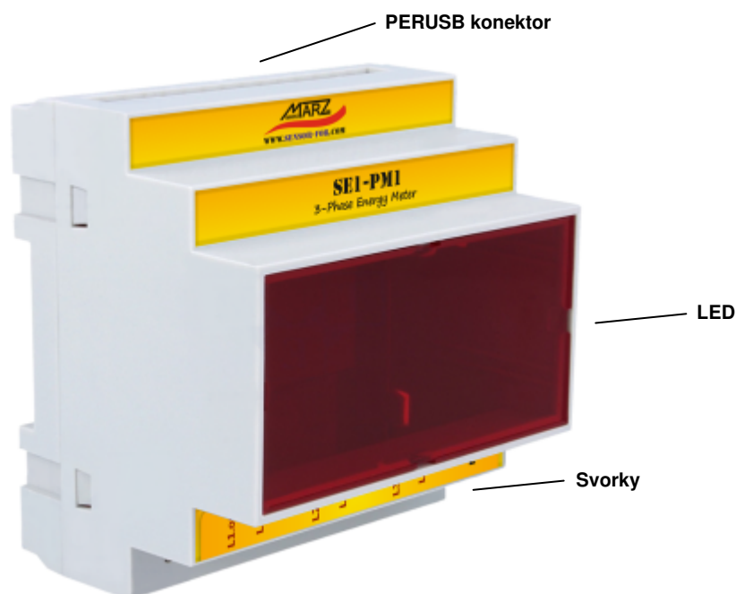
Obr. 3 Popis modulu SE1-PM1
