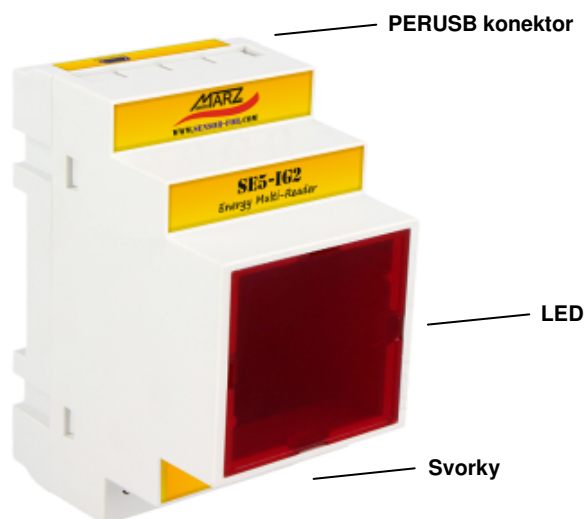
Obr. 3 Popis modulu SE5-IG2
