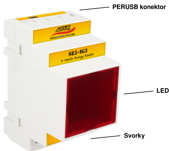
Obr. 3 Popis modulu SE5-IG3
