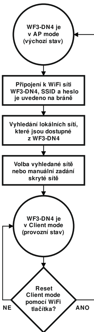
Obr. 4.1 Stavový diagram činnosti WiFi modulu
