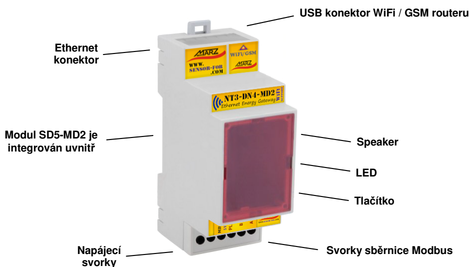
Obr. 2 NT3-DN4-MD2, popis zadní a přední strany
