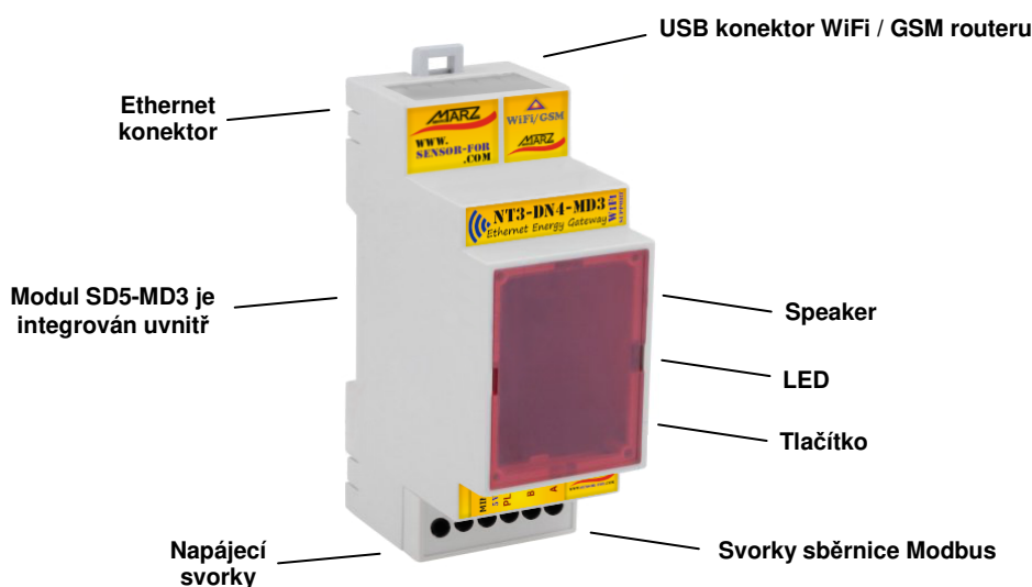
Obr. 2 NT3-DN4-MD3, popis zadní a přední strany
