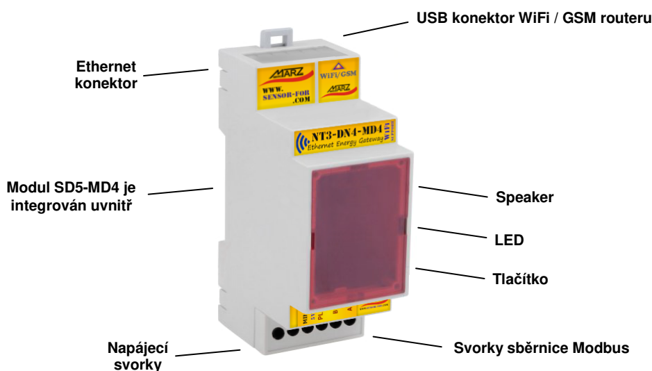
Obr. 2 NT3-DN4-MD4, popis zadní a přední strany
