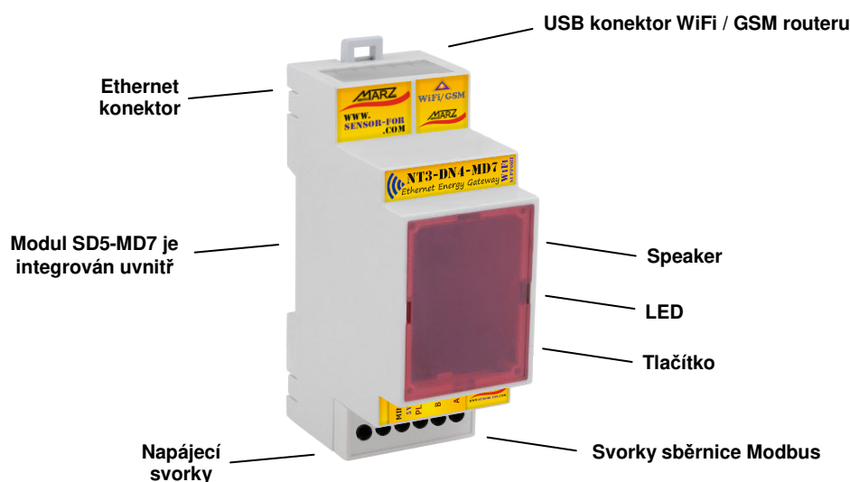
Obr. 2 NT3-DN4-MD7, popis zadní a přední strany
