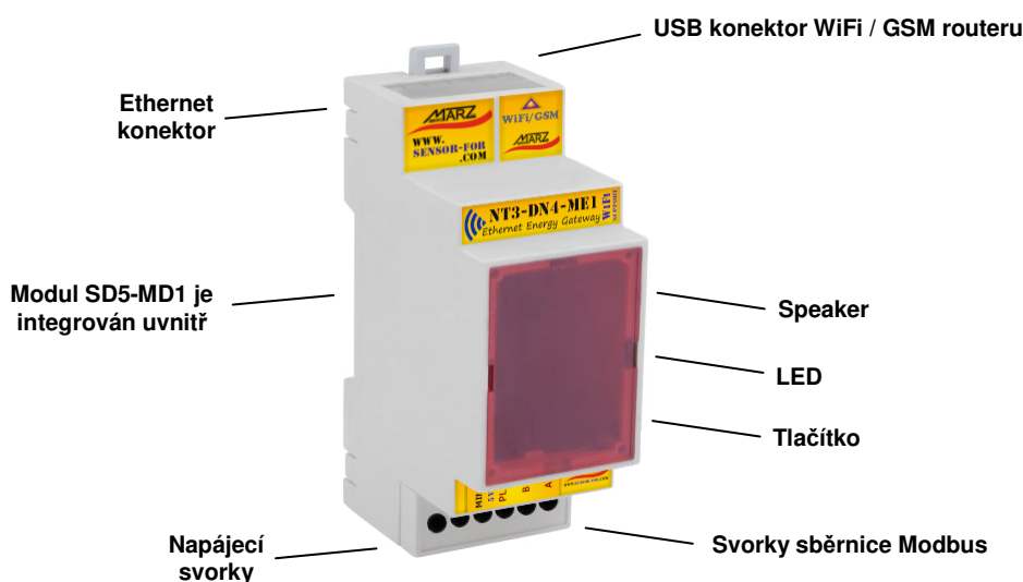
Obr. 2 NT3-DN4-ME1, popis zadní a přední strany
