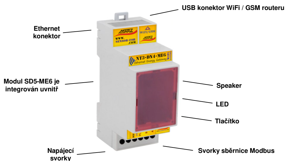
Obr. 2 NT3-DN4-ME6, popis zadní a přední strany
