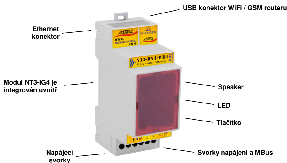
Obr. 2 NT3-DN4-WB4, popis zadní a přední strany
