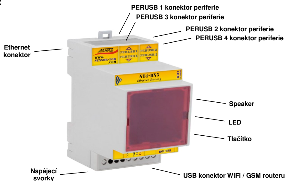
Obr. 2 NT4-DN5, popis zadní a přední strany
