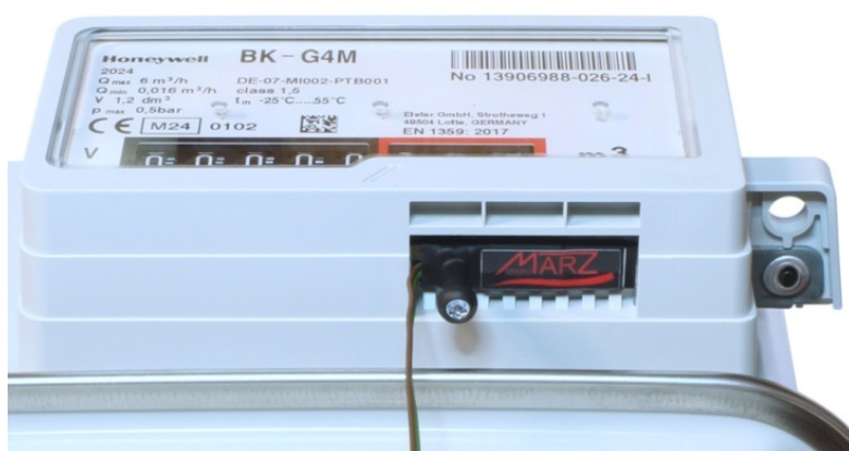
Obr. 1 Modul impulsního výstupu PU2-GS1 usazený v plynoměru BK-G4
