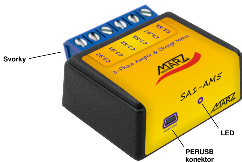
Obr. 3 Popis modulu SA1-AM5
