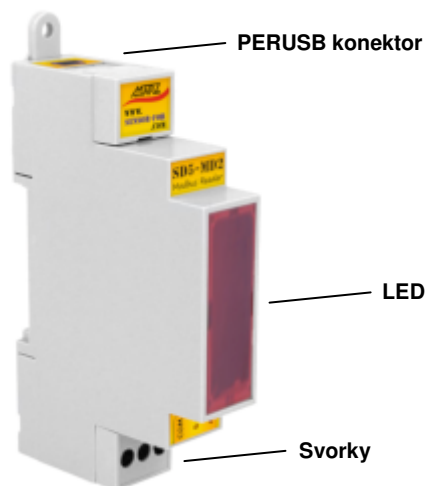
Obr. 3 Popis modulu SD5-MD2
