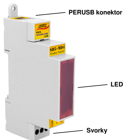
Obr. 3 Popis modulu SD5-MD4
