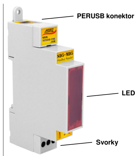
Obr. 3 Popis modulu SD5-MD5
