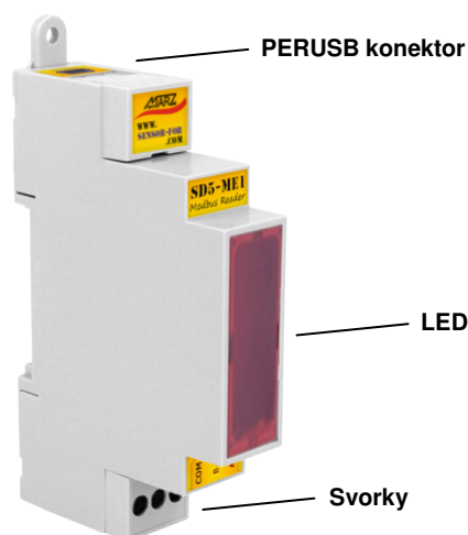
Obr. 3 Popis modulu SD5-ME1
