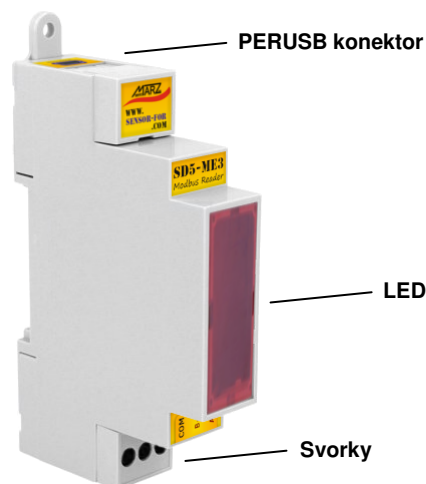
Obr. 3 Popis modulu SD5-ME3
