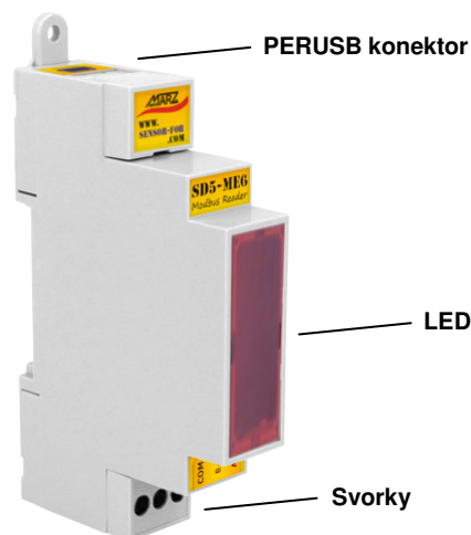
Obr. 3 Popis modulu SD5-ME6
