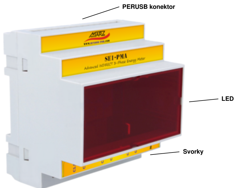
Obr. 3 Popis modulu SE1-PMA
