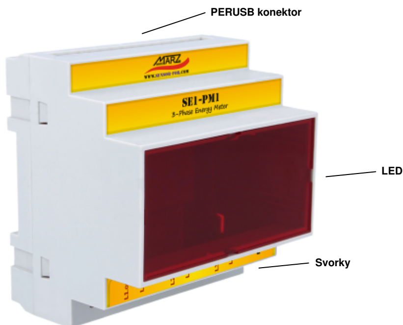
Obr. 3 Popis modulu SEI-PM1
