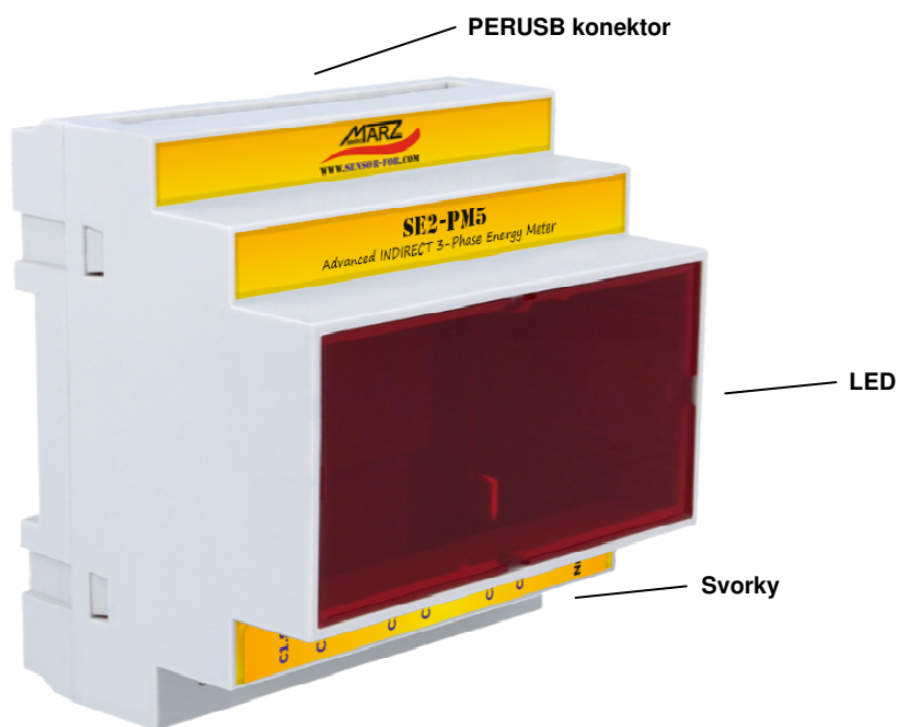
Obr. 3 Popis modulu SE2-PM5
