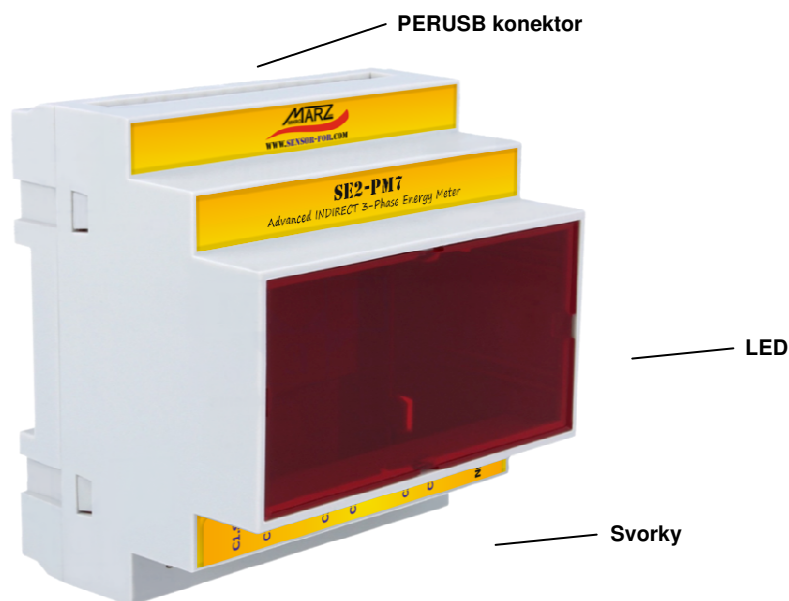
Obr. 3 Popis modulu SE2-PM7
