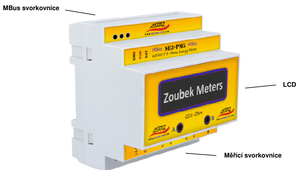
Obr. 2 Popis MBus elektroměru SE3-PM5-LCD
