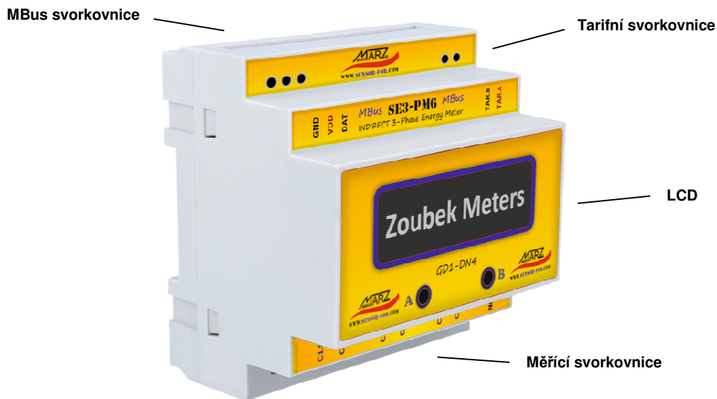
Obr. 2 Popis MBus elektroměru SE3-PM6-LCD
