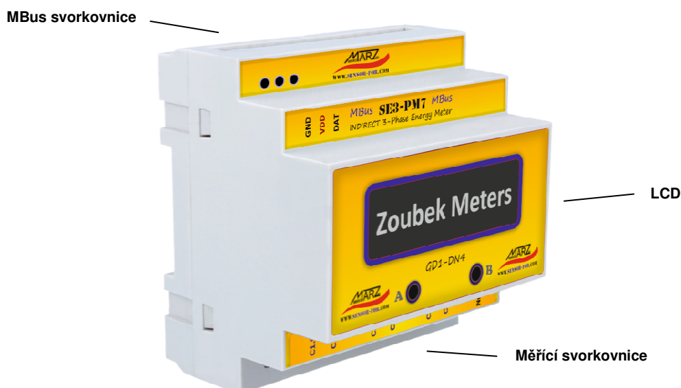
Obr. 2 Popis MBus elektroměru SE3-PM7-LCD
