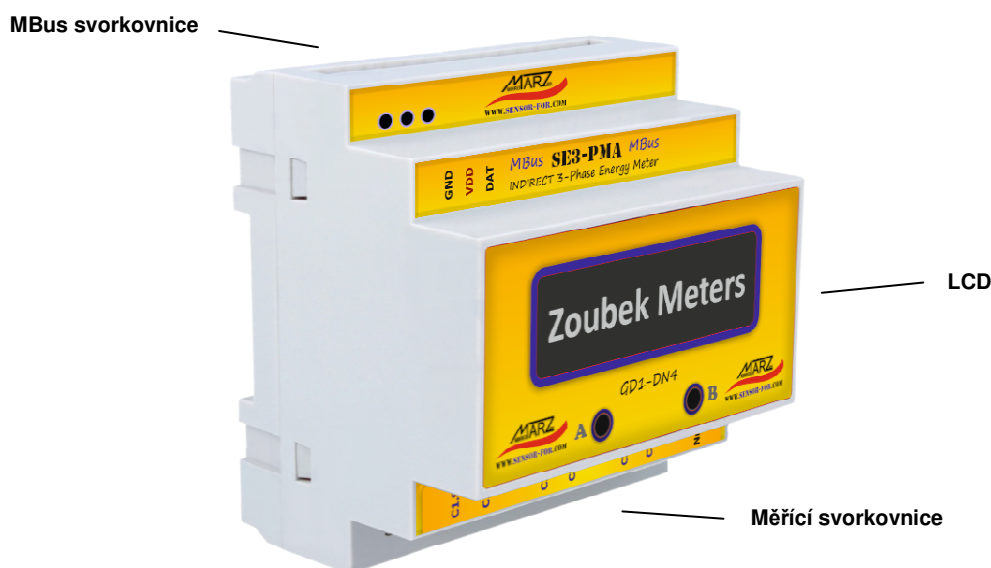
Obr. 2 Popis MBus elektroměru SE3-PMA-LCD
