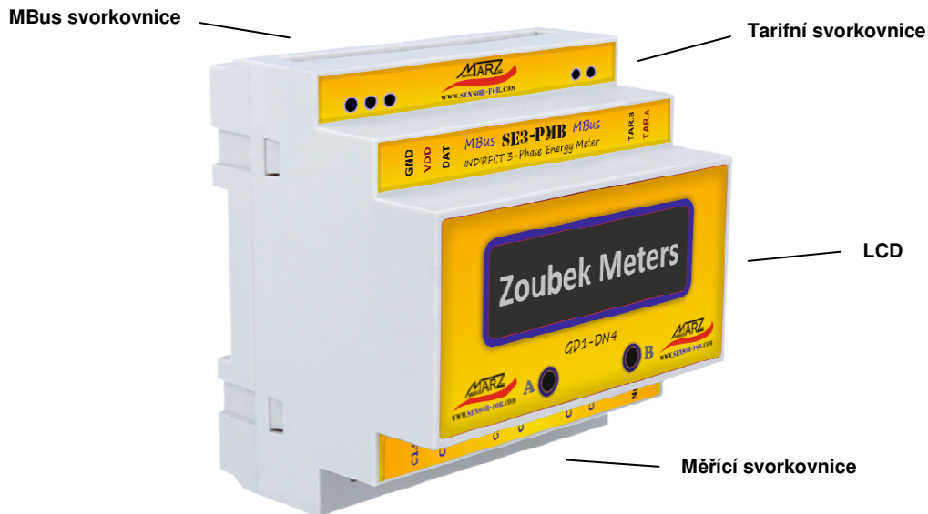
Obr. 2 Popis MBus elektroměru SE3-PMB-LCD
