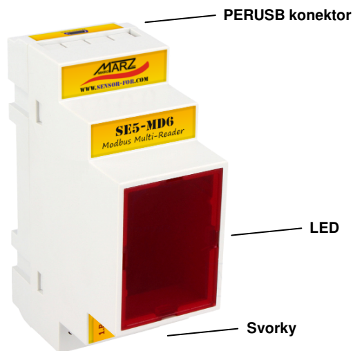
Obr. 3 Popis modulu SE5-MD6
