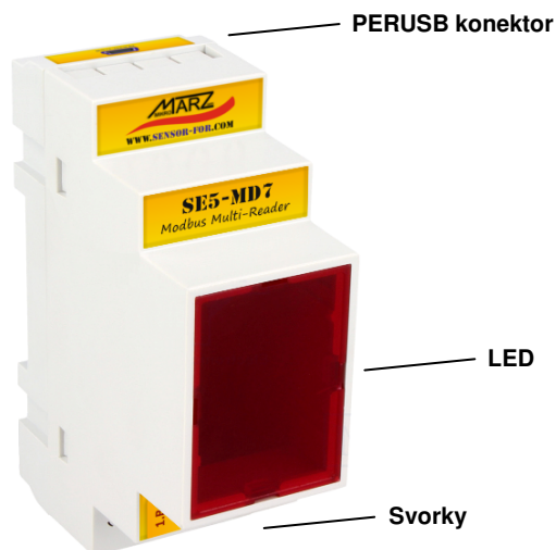
Obr. 3 Popis modulu SE5-MD7
