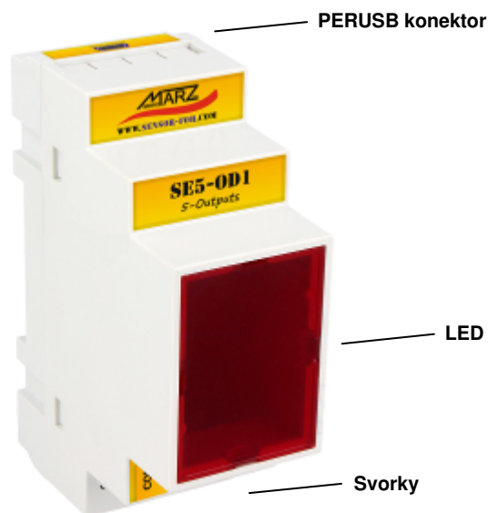
Obr. 3 Popis modulu SE5-OD1
