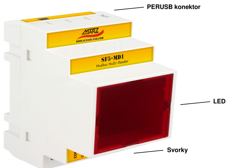
Obr. 3 Popis modulu SF5-MD1
