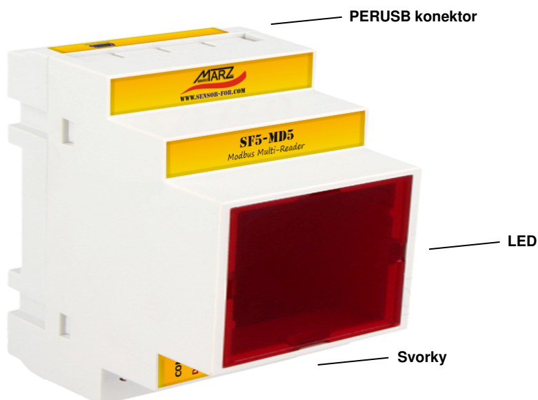
Obr. 3 Popis modulu SF5-MD5
