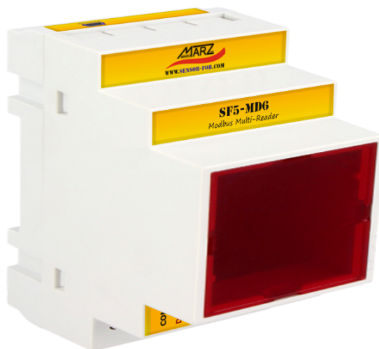
Obr. 1 Modbus čtečka elektroměrů SF5-MD6
