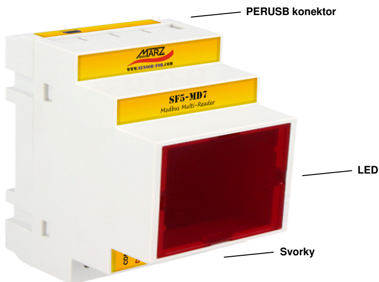
Obr. 3 Popis modulu SF5-MD7
