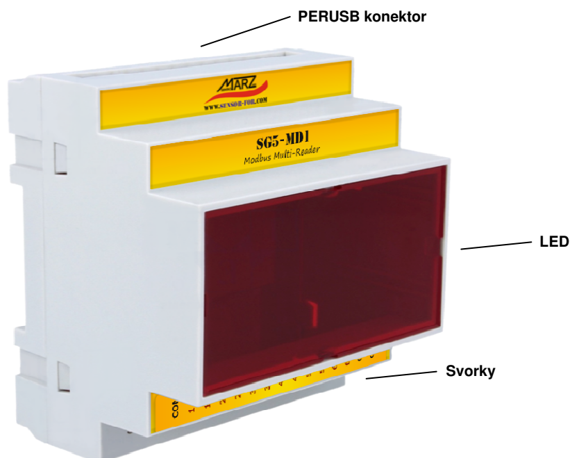
Obr. 3 Popis modulu SG5-MD1
