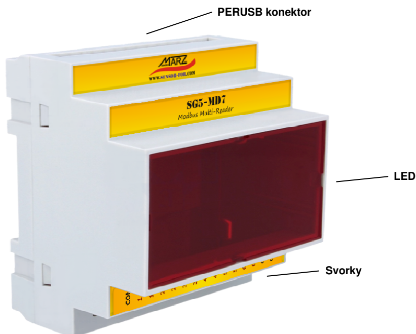
Obr. 3 Popis modulu SG5-MD7
